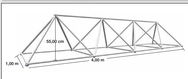
Χωροδικτύωμα
